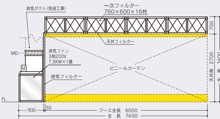
側面図
