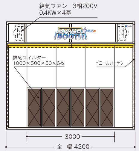
正面図
