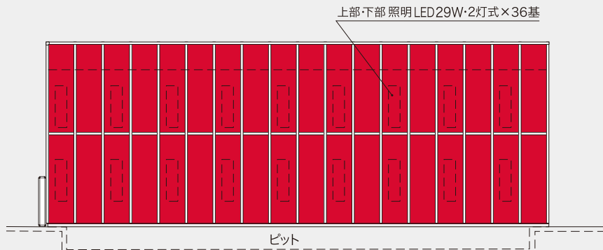
側面図
