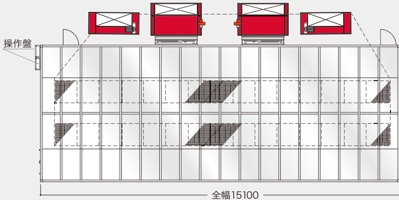
平面図
